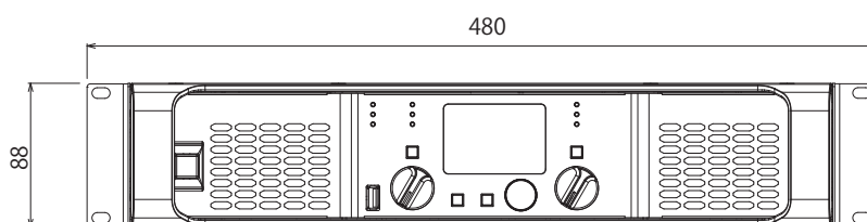
正面図
