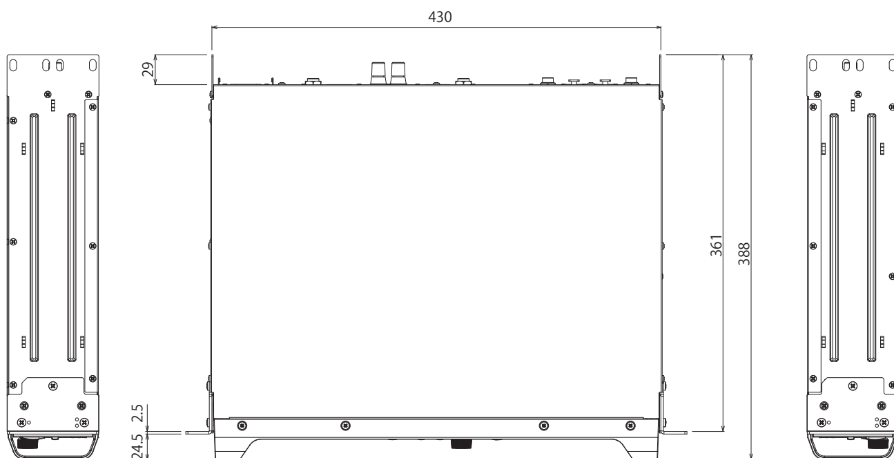
左側面図
