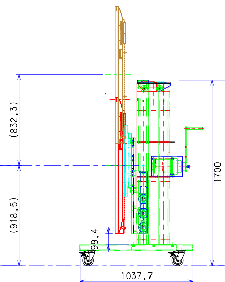
ウィンチ式 1 段昇降スタンド
