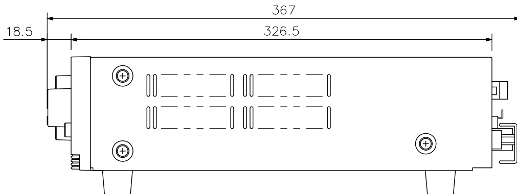
側面図
