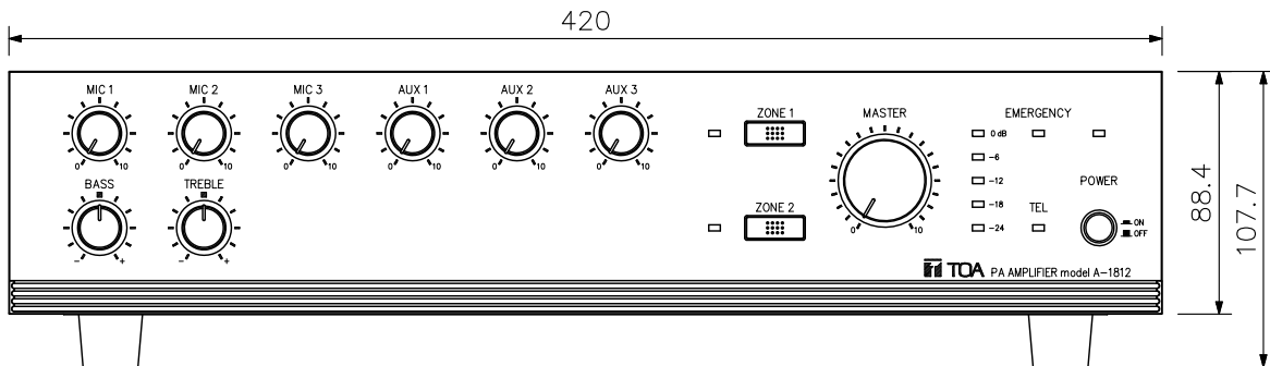
正面図
