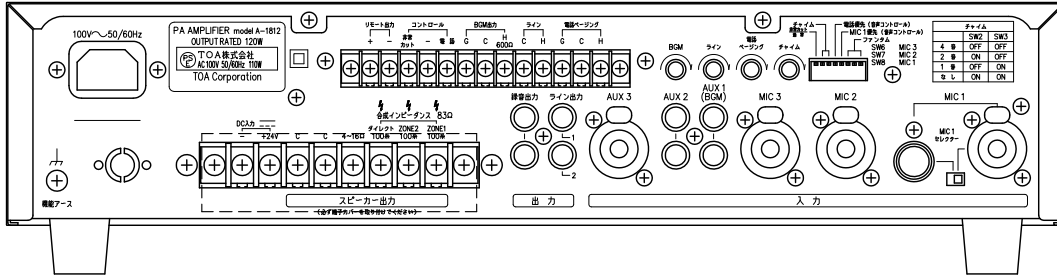
背面図
